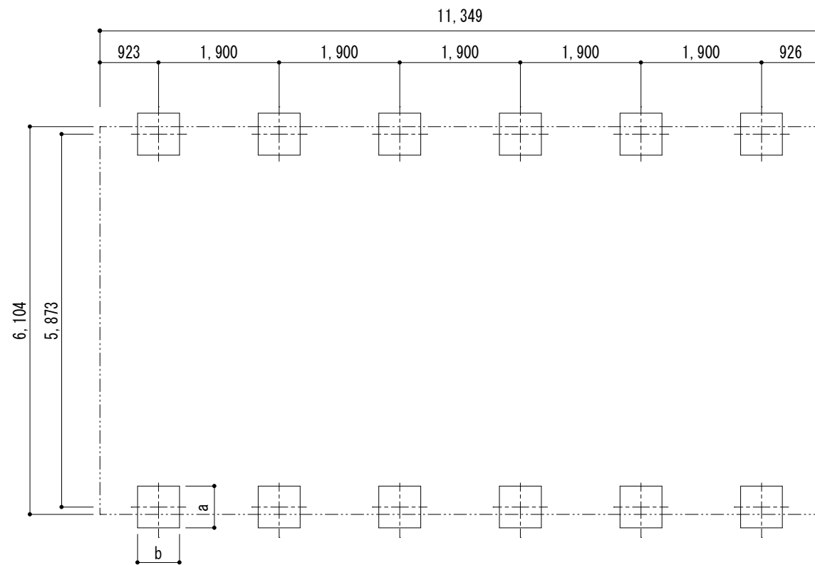
■基礎配置図
